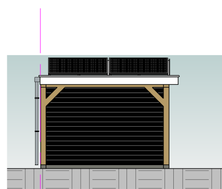
veranda A Linkergevel
